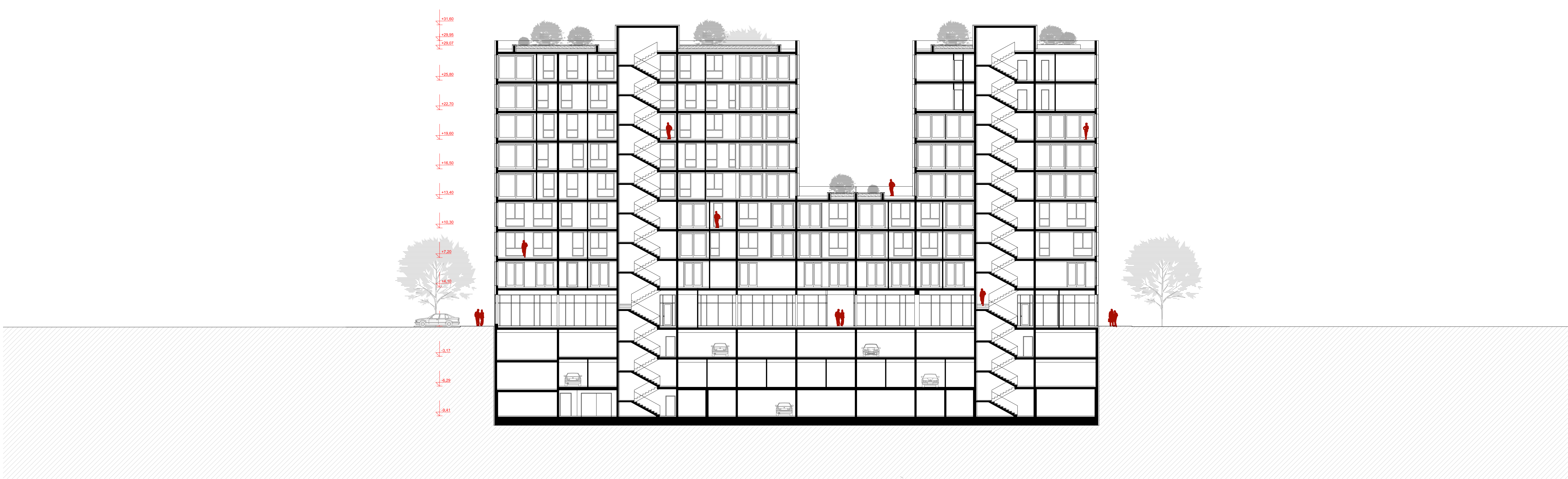
PRESJEK C-C M 1:200
