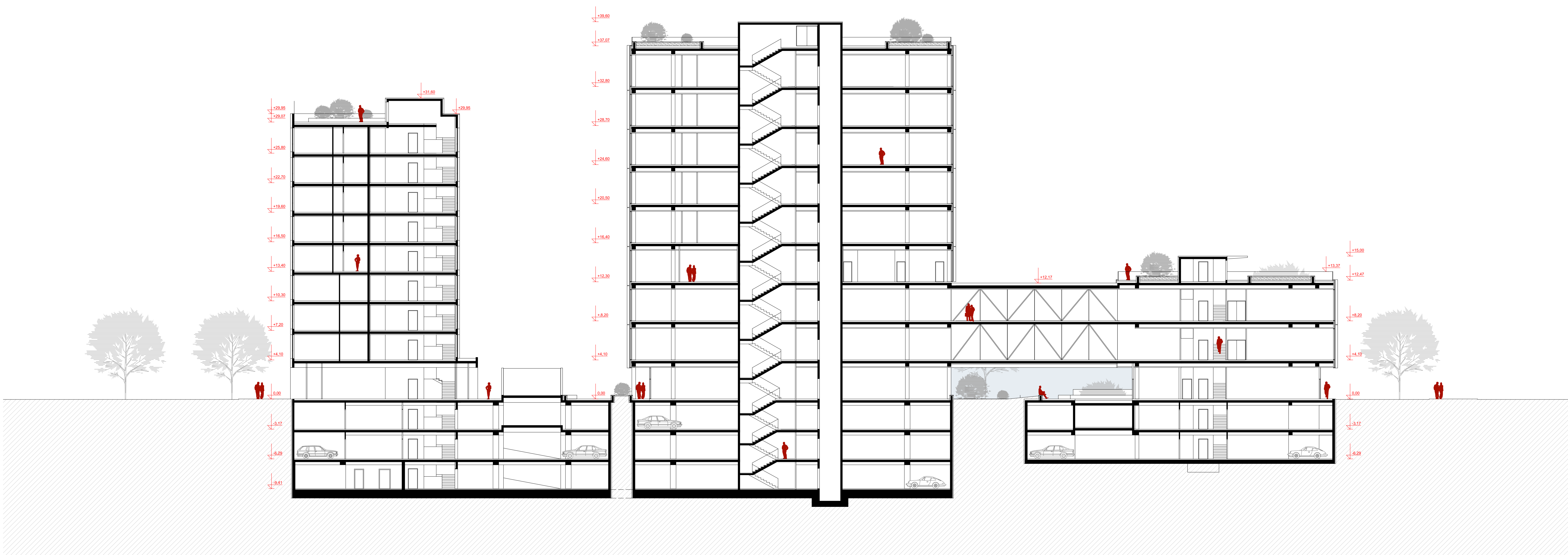
PRESJEK B-B M 1:200
