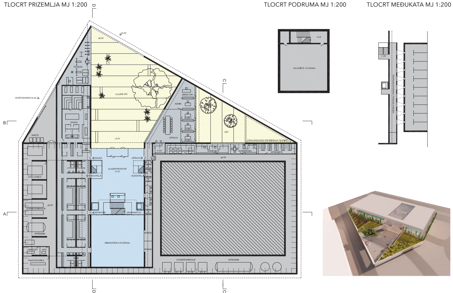
TLOCRT PRIZEMLJA MJ 1:200
