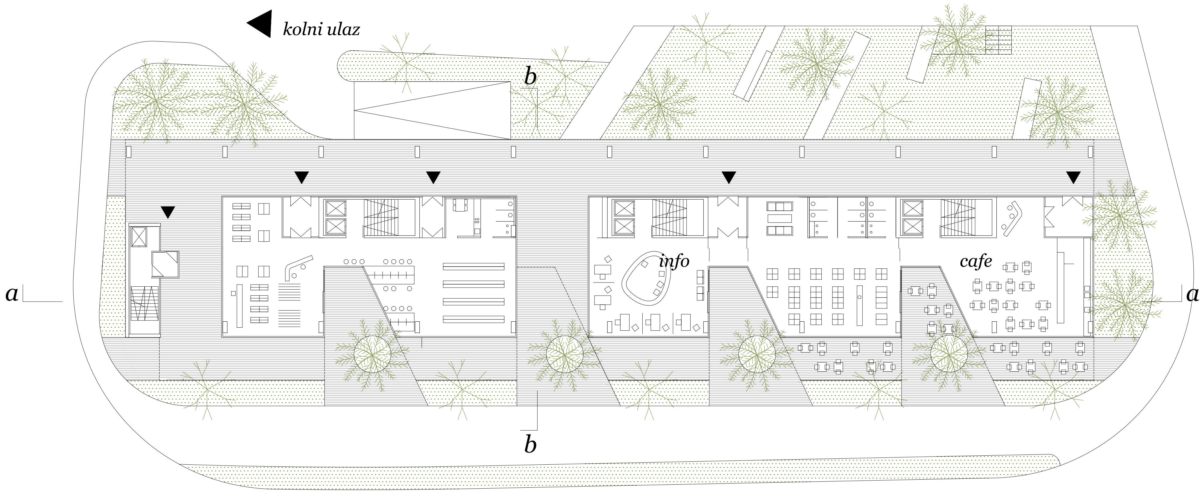
prizemlje 1:200
