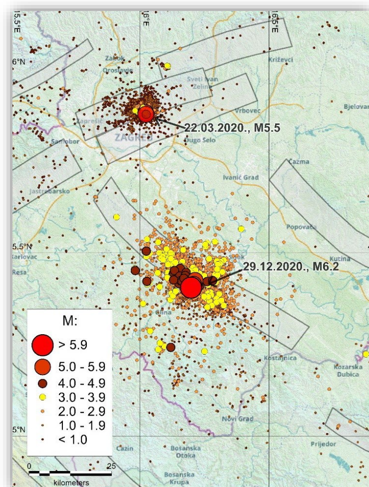
Karta potresnih središta za razdoblje između potresa u ožujku i potres u prosincu 2020.
