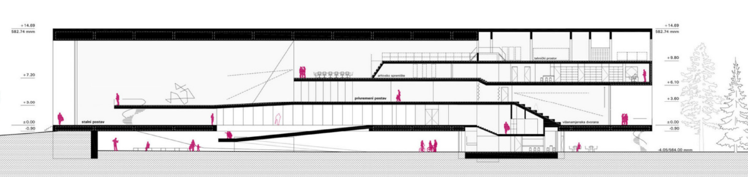
PRESJEK d-d
