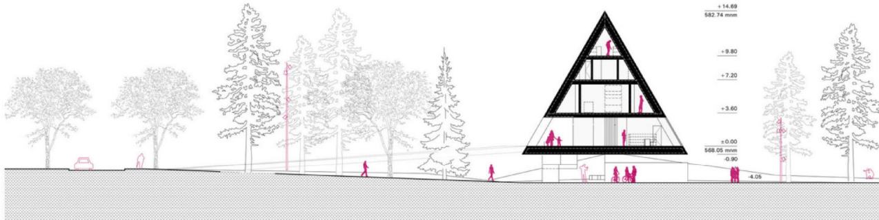
PRESJEK b-b
