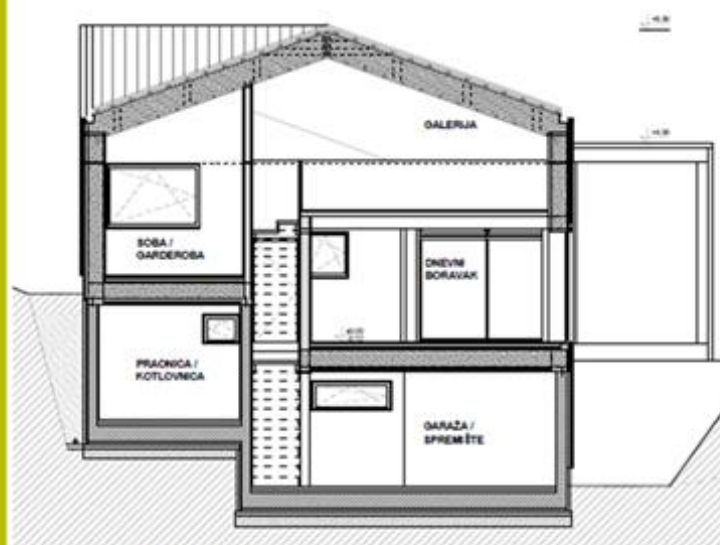
PRESJEK 1 / M 1:100
