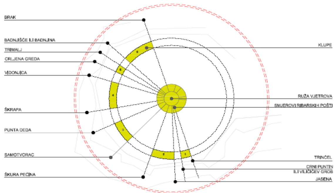
PRIKAZ SMJEROVA I POZICIJA RIBARSKIH POŠTI KOJI DEFINIRAJU VELIČINU I IZGLED KLUPA
