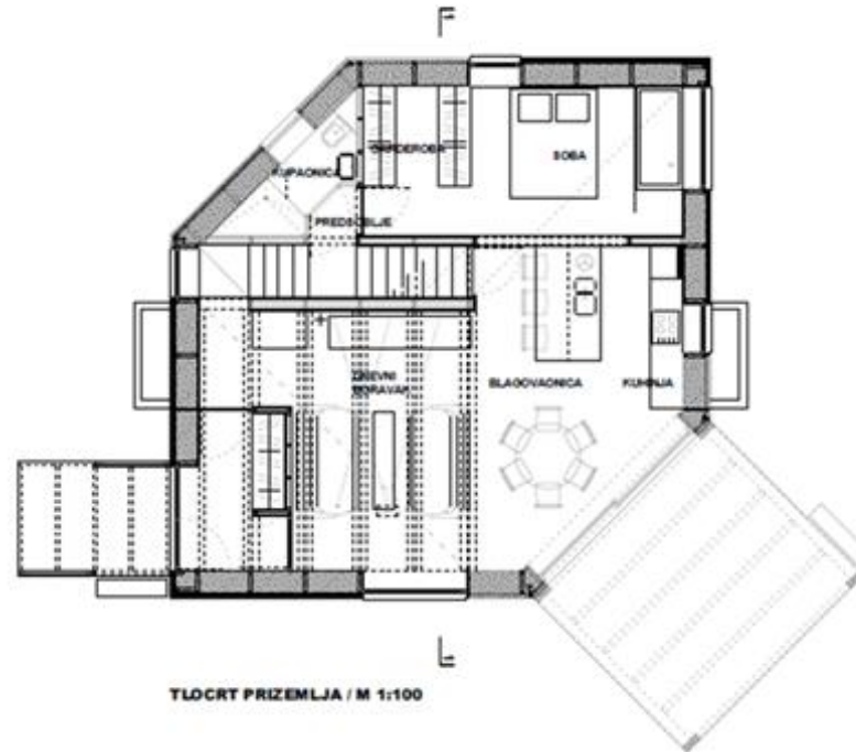
TLOCRT PRIZEMLJA / M 1:100
