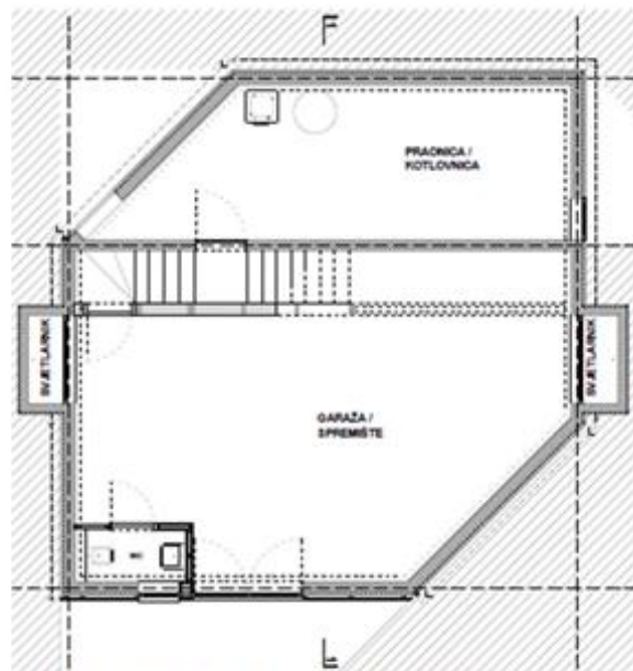
TLOCRT PRETEŽITO UKOPANE ETAŽE / M 1:100
